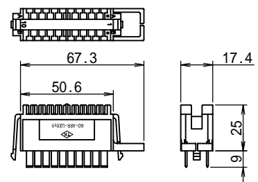
60-ARR-Uスリット(オプション)
